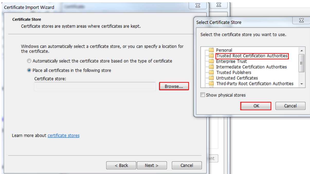
Rys. 4. Wybór konteneru Zaufane główne urzędy certyfikujące
